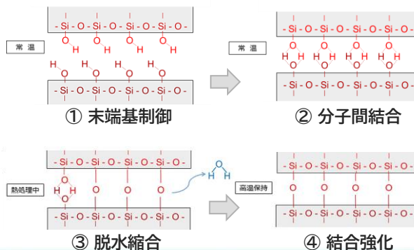
石英ガラス基材 製品構造 (特許取得済)
