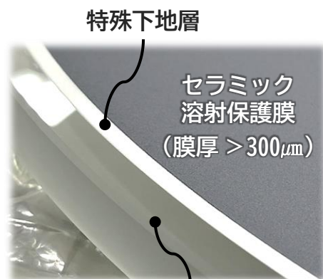
石英ガラス基材 製品構造 (特許取得済)
